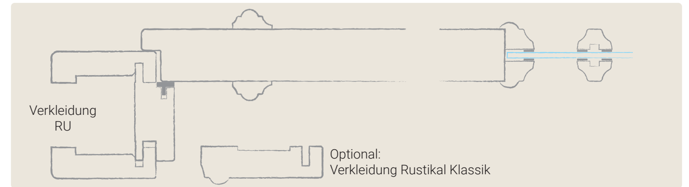
Profil S1
